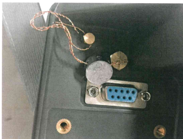
Рисунок 2 - Место пломбировки весов
