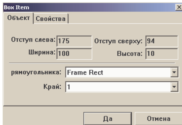
Рисунок 9.7 – Параметры прямоугольника
